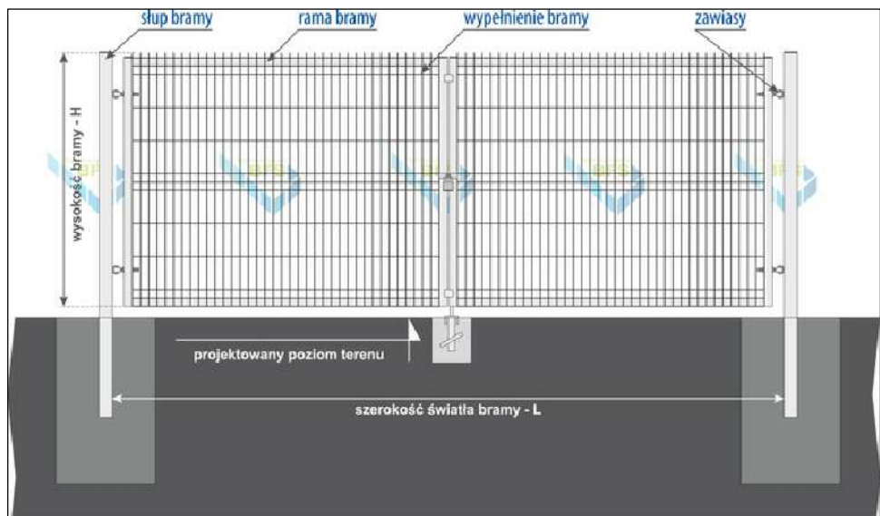
Widok bramy rozwiernej systemowej
