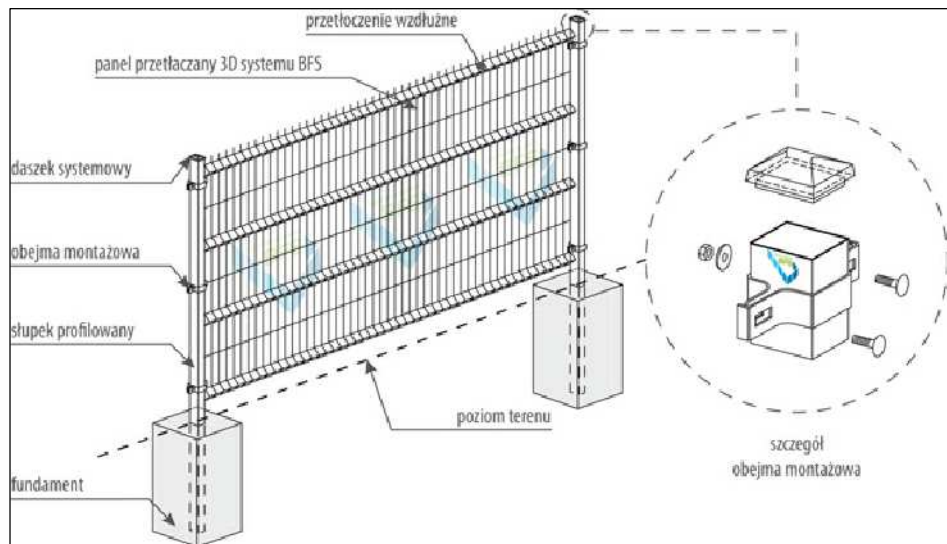
Widok panela systemowego z fundamentem
