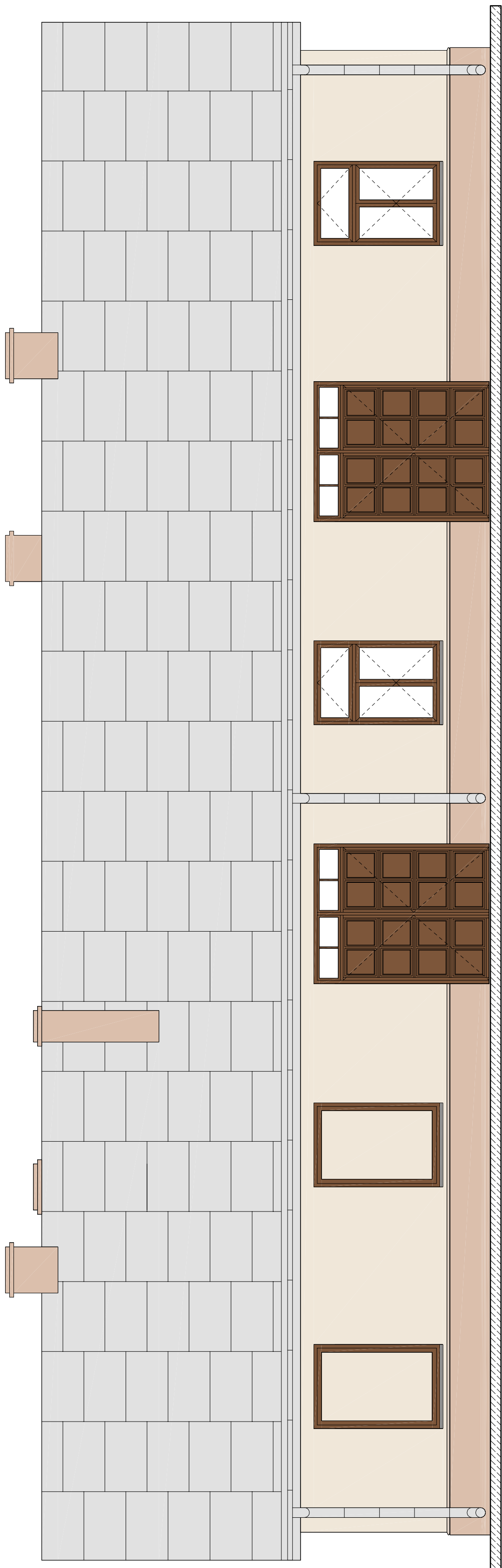
ELEWACJA POŁUDNIOWA SKALA 1:100
