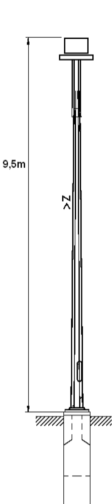
SŁUP STALOWY SZEŚCIOKĄTNY OCYNKOWANY FUNDAMENT F150/200
